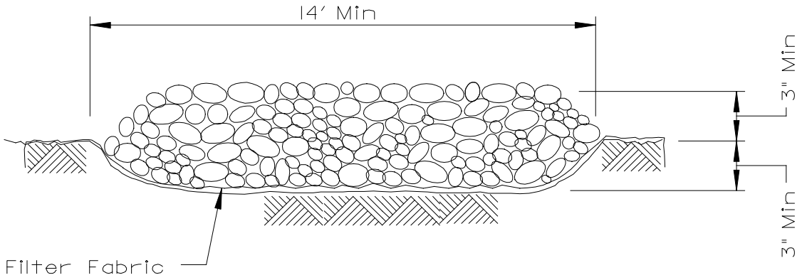
SECTION A-A
